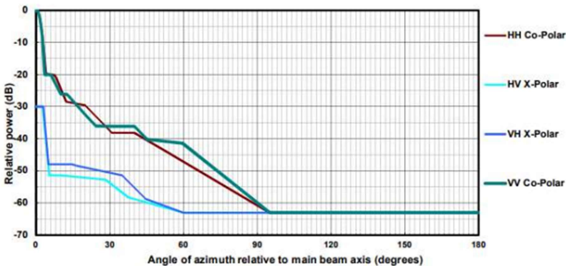
Compliance To ETSI EN 302 217-4-2V 1.5.1 Range1, Class3
